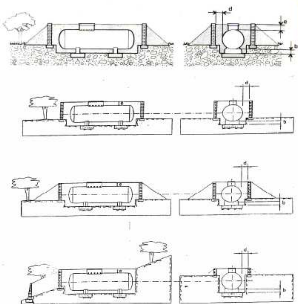
FIGURA 5. Tanques semienterrados
