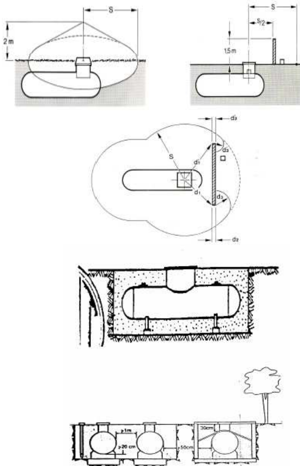
FIGURA 4. Tanques enterrados
